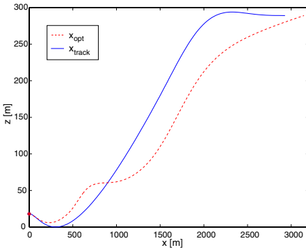
Fig. 7. Trajectories in longitudinal plane
